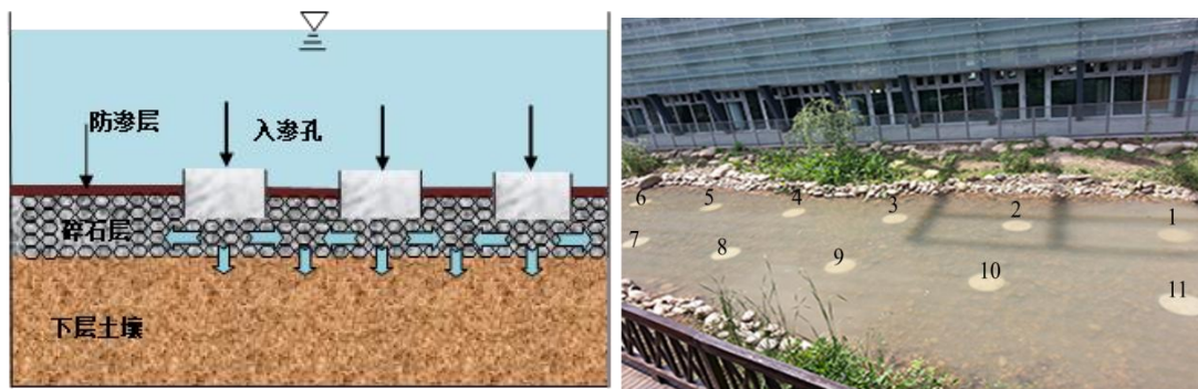
图 F4-7 城市最佳实践区北区荷花池下渗改造（左：示意图；右：实景图）
