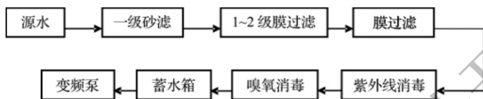
图 6.5.3 管道直饮水水处理工艺流程
