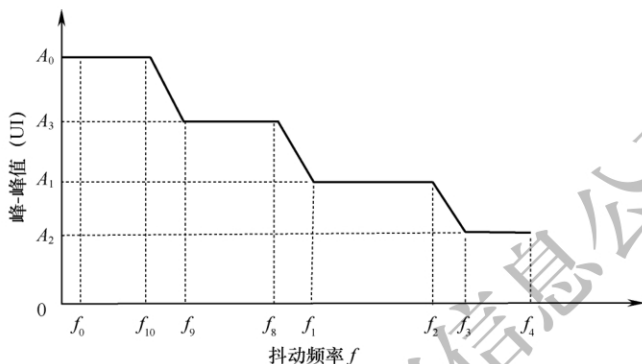
图 8.2.6-2 STM-64 输入抖动容限图形模板
