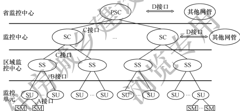
图 8.0.2 动力及环境监控系统网络结构
