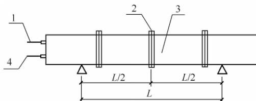
图 A.3.1 试验用风管
