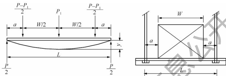
图 4.2.3 吊架载荷分布图
