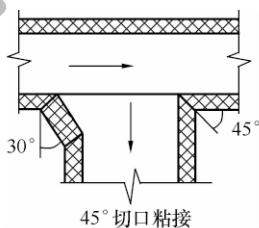
图 4.5.6 主风管上直接开口连接支风管方式
