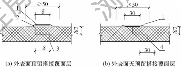
图 3.6.2-1 玻璃纤维复合板拼接
