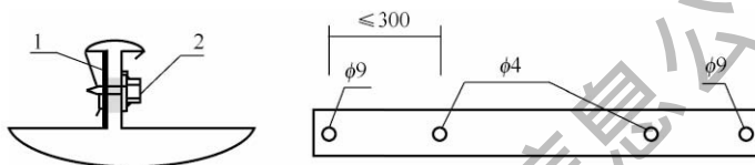
图 4. 4. 3 薄钢板法兰板条加固示意图
