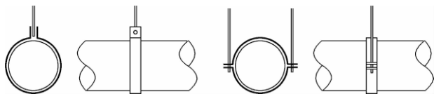
图 4.2.14 柔性风管卡箍安装
