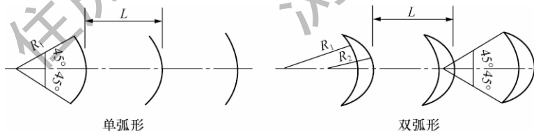
图 3.11.2-2 导流片形式
