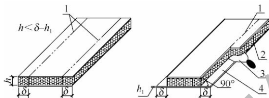
图 3.6.4-1 风管侧板阶梯线切割示意图
