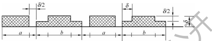
图 3.6.2-2 玻璃纤维复合板风管 90°梯形槽口
