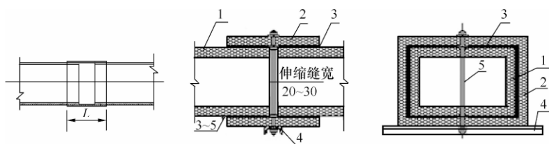
图 3.6.4-9 伸缩节构造示意图
