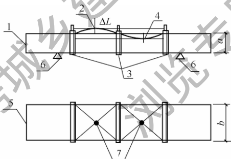
图 A.5.2 管壁变形量试验图
