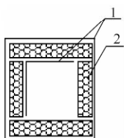
图 3.6.3 四片 90° 组合方式
