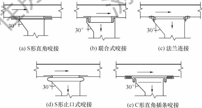
图 4.4.7 支风管与主风管连接方式
