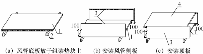
图 3.6.4-6 风管组装示意图
