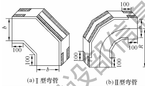
图 3.6.4-4 90°弯管放样下料示意图
