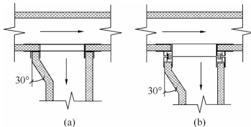
图 4.3.8 主风管与支风管 90^\circ 连接示意图
