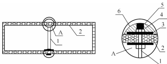
图 3.6.4-8 隔热风管内支撑加固示意图
