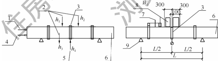
图 A.4.1 风管测试装置图
