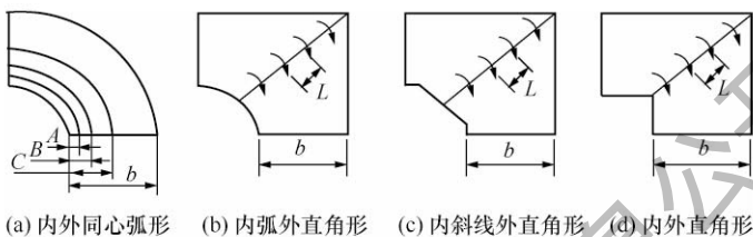
图 3.11.2-1 矩形弯管示意图
