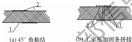
图 3.6.1-1 风管板材拼接方式
