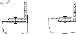
图 4.7.3 柔性风管与角钢法兰的连接
