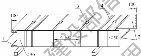
图 3.6.4-7 风管捆扎示意图
