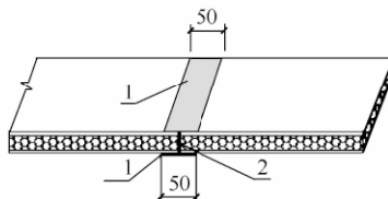
图 3.6.4-3 复合板拼接方法示意图
