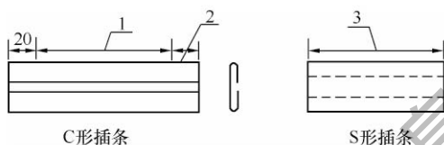
图 3.2.4 C 形、S 形插条示意图
