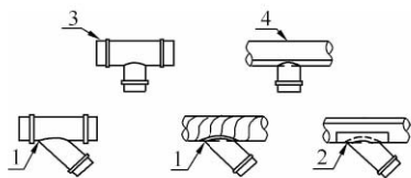
图 3.11.5 三通连接形式
