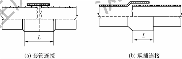
图 4.5.5 硬聚氯乙烯、聚丙烯（PP）风管连接
