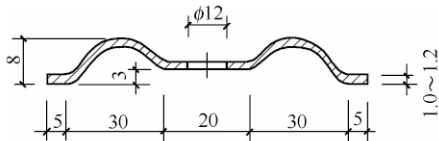
图 3.6.2-4 波纹槽形加固件
