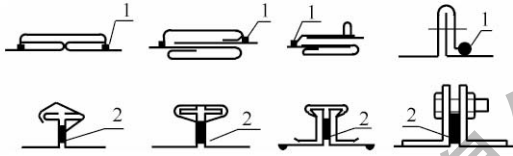
图 4.3.5-1 矩形风管管段连接的密封
