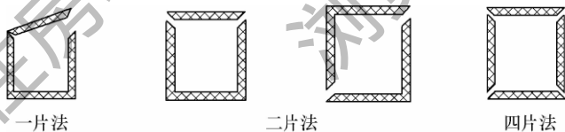
图 3.6.1-2 矩形风管 45°角组合方式
