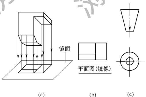
图 10.1.2 镜像投影法
