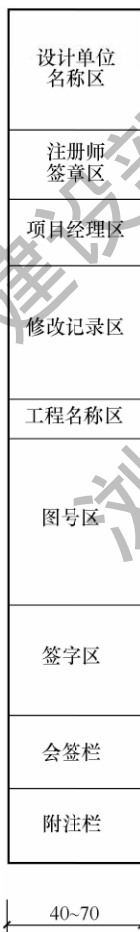
图 3.2.2-1 标题栏（一）
