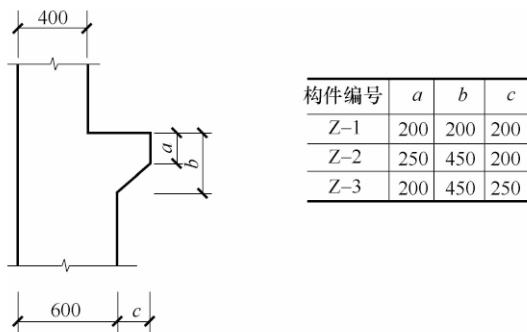
图 11.7.6 相似构配件尺寸表格式标注方法
