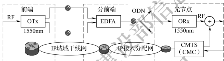
图 5.4.3-1 单级光纤链路 HFC 方式下 CMTS 前端部署系统框图
