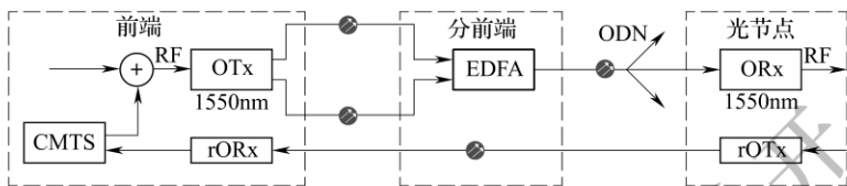
图 5.4.3-1 单级光纤链路 HFC 方式下 CMTS 前端部署系统框图
