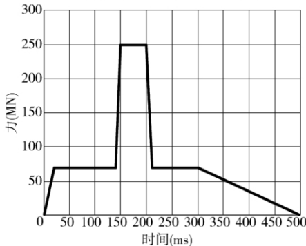
图 C. 2. 2 飞机撞击荷载时程曲线
