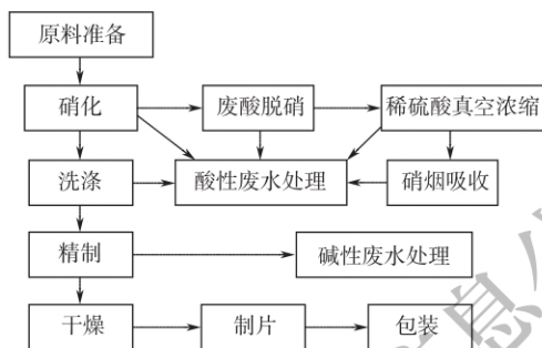
图 2.2.1 梯恩梯生产工艺流程图
