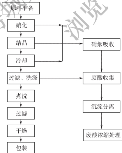
图 2.2.3 黑索今生产工艺流程图
