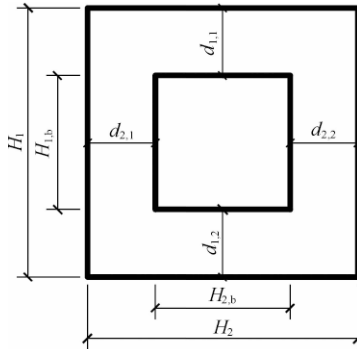
图 P. 5.1 矩形钢构件的主控尺寸
