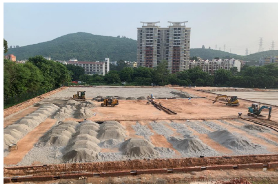
安装滤水管、铺设碎石
